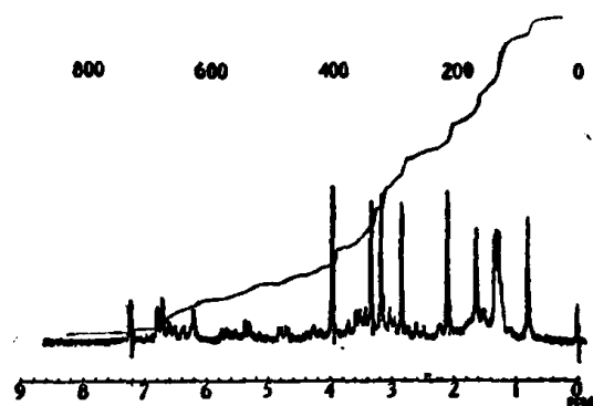
图 2 M-1 晶的核磁共振谱 (100 兆赫)
