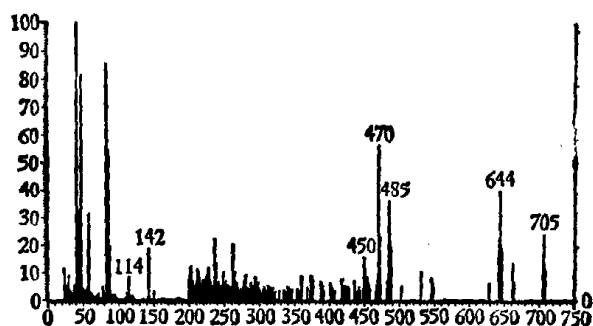
图 3 M-2 晶质谱 (70eV, 直接进样)
