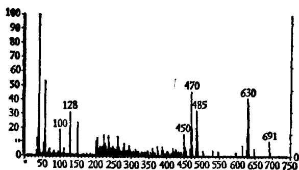
图 1 M-1 晶质谱 (70eV, 直接进样)
