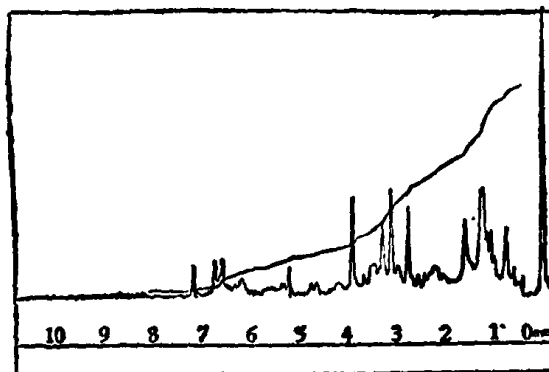
图 4 M-2 晶核磁共振谱 (100 兆赫)
