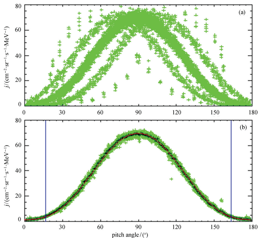
图 1 磁赤道面上 RBSP A 卫星观测所得 E = 208 MeV, L = 1.39 组投掷角数据分布. (a) 未经处理的投掷角数据分布, (b) 处理后的投掷角数据分布及拟合结果
