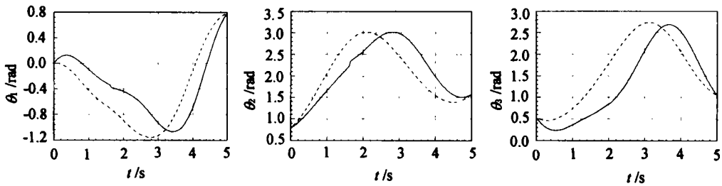
图 4 载体姿态和机械臂关节角优化轨迹
