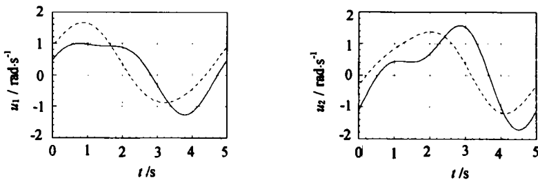
图 5 最优控制输入规律
