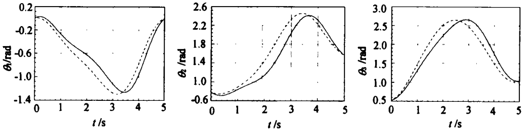
图 2 载体姿态和机械臂关节角优化轨迹
