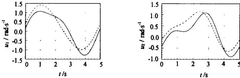
图 3 最优控制输入规律
