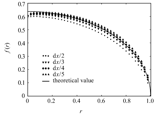
图 2 不同栅格位移得到的结果比较
