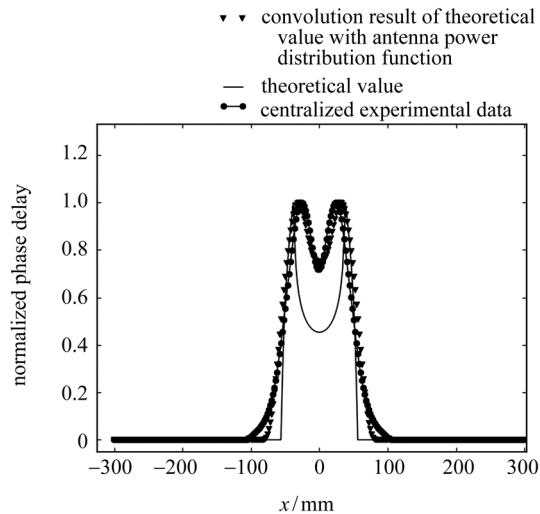
图 10 对称化后的测量值与理论值的对比
