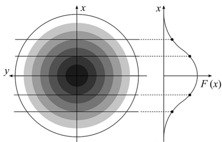
图1 径向分布函数 f(r) 与 Abel 变换关系
