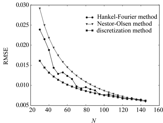
图4 均方根误差与 N 之间的关系
