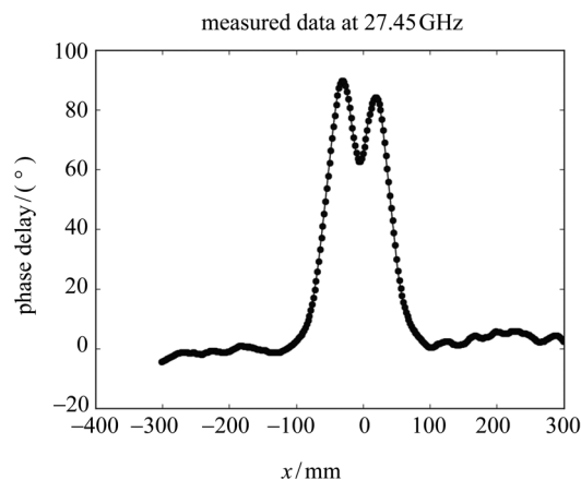
图 8 实验测量得到的相移数据 ( f_{\text{req}} = 27.45 \text{ GHz} )
