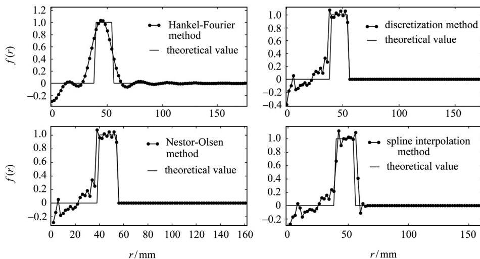
图 9 对实验数据进行 Abel 逆变换的结果
