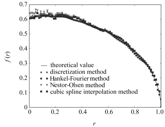
图 6 进行平滑处理后的 Abel 逆变换结果
