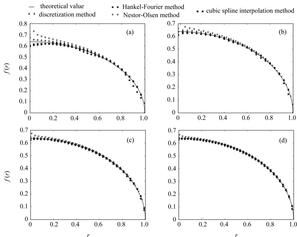
图3 四种 Abel 逆变换算法比较 (a) N = 30 , (b) N = 50 , (c) N = 100 , (d) N = 150
