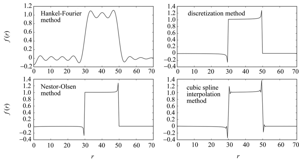
图 7 四种方法反演不连续分布函数
