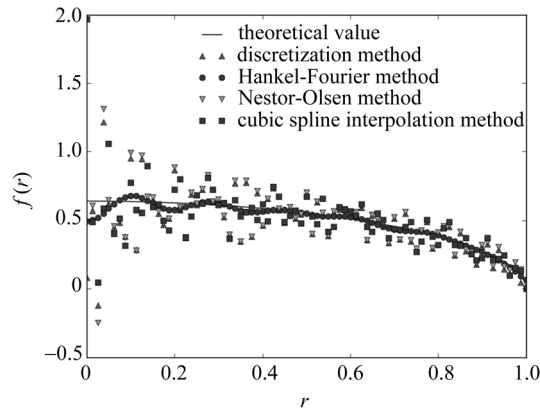
图 5 加 5% 噪声后的 Abel 逆变换结果
