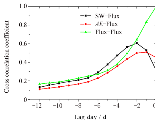
图 6 太阳风速度、地磁 AE 指数与 GEO 轨道相对论电子通量以及相对论电子通量自身之间的线性相关关系
