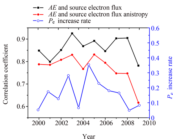
图 7 Model-1 较持续模型的预报效率提升比例, AE 指数对数值与源电子通量对数值和通量各向异性对数值的相关性
