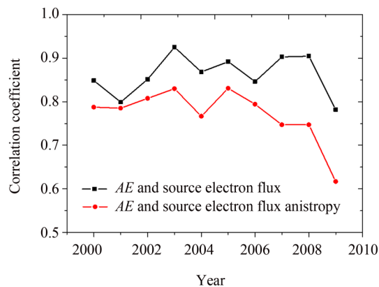
图 5 地磁 AE 指数、源电子通量及源电子通量各向异性的线性相关性
