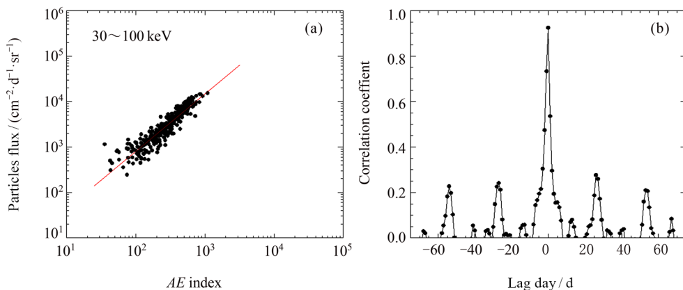
图 3 2003 年源电子通量与地磁 AE 指数的散点分布 (a) 及相关性 (b)
