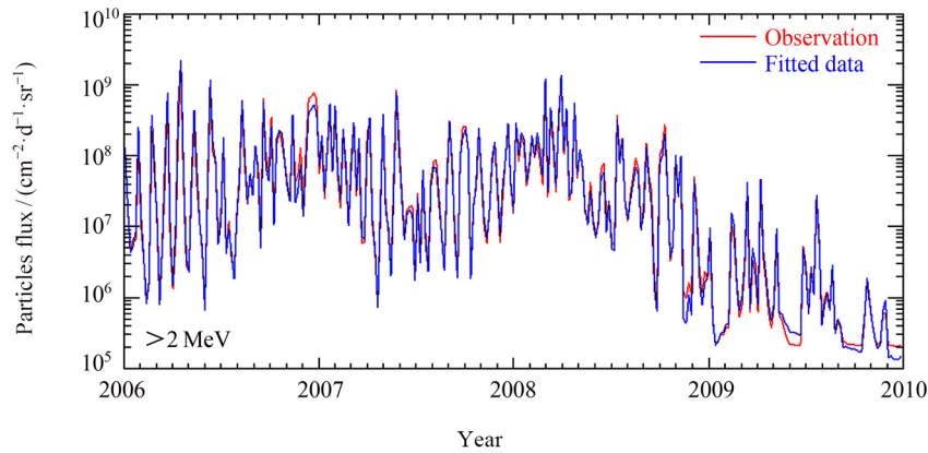
图 2 2006—2009 年 GOES 卫星观测的大于 2 MeV 相对论电子通量和拟合后的通量
