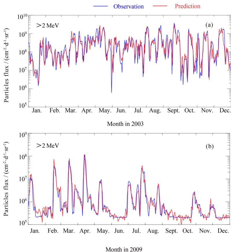
图9 2003 和 2009 年 Model-2 预报结果与观测值对比
