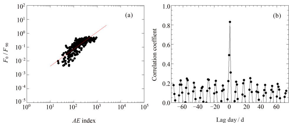
图 4 2005 年源电子通量各向异性程度和地磁 AE 指数的散点分布 (a) 及相关性 (b)
