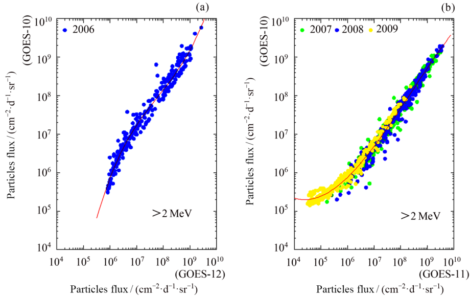
图 1 不同年份 GOES-10 和 GOES-12 (a) 及 GOES-10 和 GOES-11 (b) 卫星的观测数据
