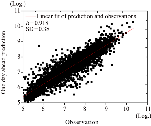
图 8 2000—2009 年大于 2 MeV 相对论电子观测值对数值和提前一天预测值对数值
