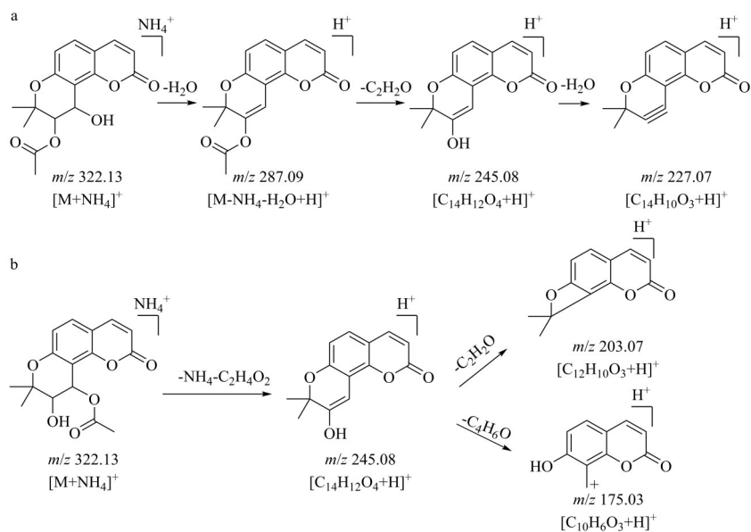
图 3 (a)前胡香豆素 B 和(b)前胡香豆素 C 可能的裂解途径
