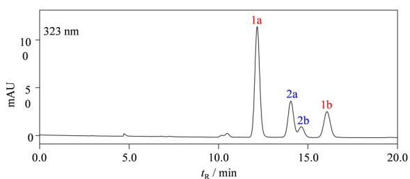
图 7 化合物 1 和 2 的对映体拆分色谱图
