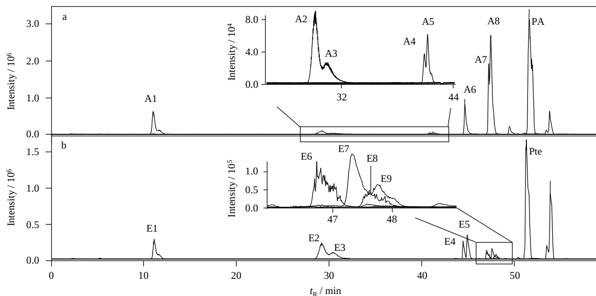
图 1 HLMs 中(a)(+)-PA 和(b)(+)-Pte 代谢产物的提取离子流图
