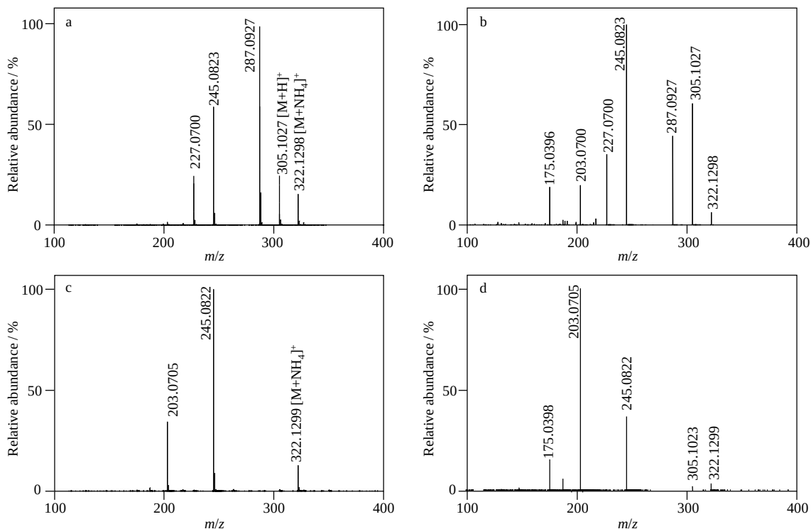
图 2 前胡香豆素 B 的 (a) MS 1 和 (b) MS 2 质谱图以及前胡香豆素 C 的 (c) MS 1 和 (d) MS 2 质谱图
