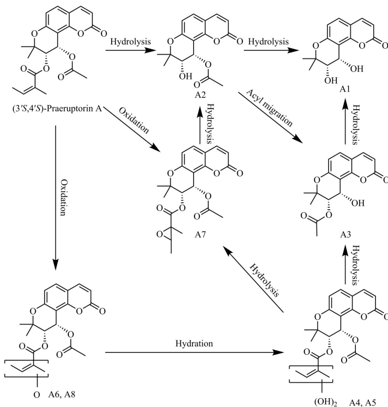
图 4 (+)-PA 在 HLMs 中可能的代谢途径
