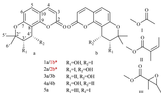
图 6 角型吡喃香豆素 1-5 的化学结构
