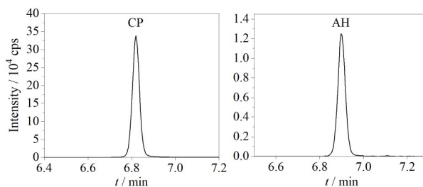
图 8 阳性马尿样品中 CP 和 AH 的色谱图
