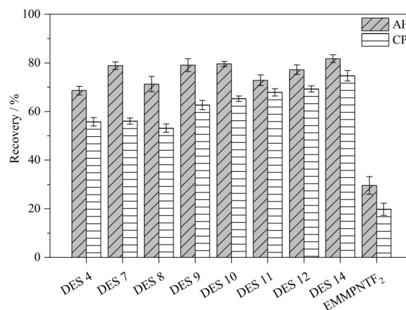
图 2 8 种 IL-DES 和 EMMPNTF_2 对马尿中 AH 和 CP 萃取率的影响 ( n=3 )
