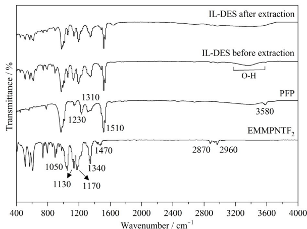
图 6 萃取后 IL-DES、萃取前 IL-DES、PFP 和 EMMPNTF 2 的红外光谱图
