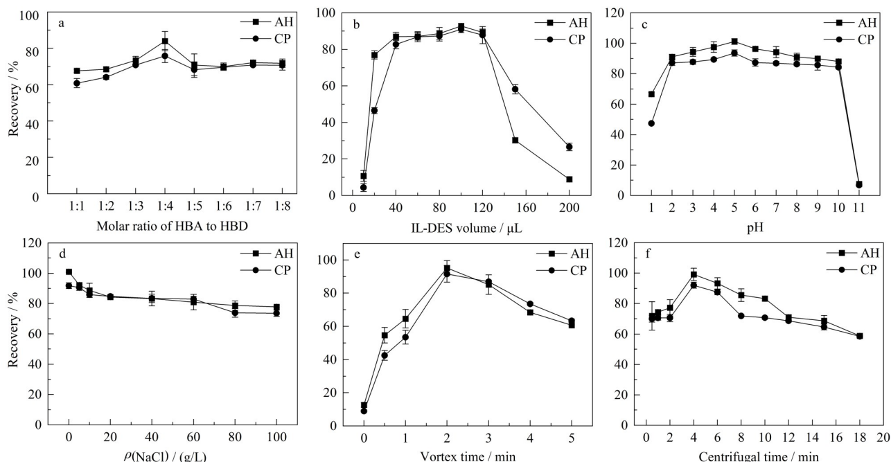
图3 (a)HBA与HBD物质的量之比、(b)IL-DES用量、(c)pH、(d)NaCl质量浓度、(e)涡旋时间和(f)离心时间对马尿中AH和CP萃取率的影响( n=3 )
