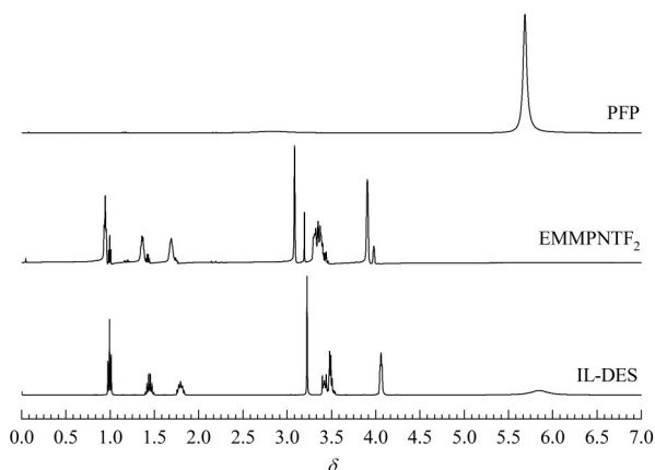
图 5 PFP,EMMPNTF 2 和 IL-DES 的核磁共振氢谱图
