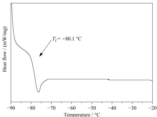
图 4 IL-DES(DES 14,下同)的差示扫描量热图
