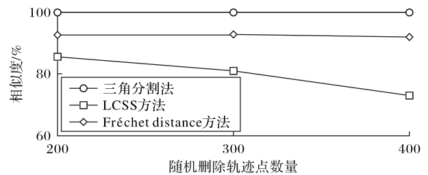
图4 轨迹点随机缺失的轨迹相似度量变化
