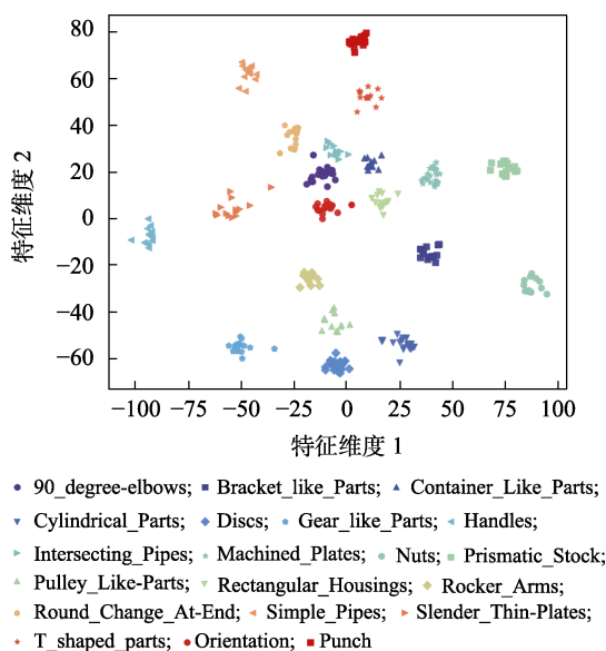
图 10 基于 t-SNE 的融合特征可视化结果
