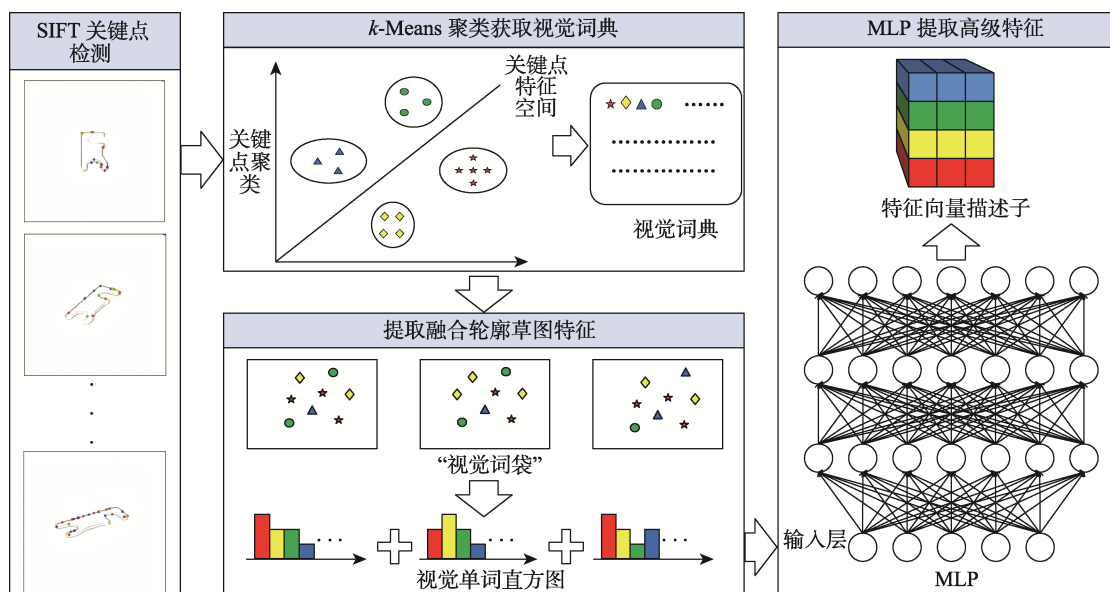
图 4 基于 BOVW 的局部特征提取过程
