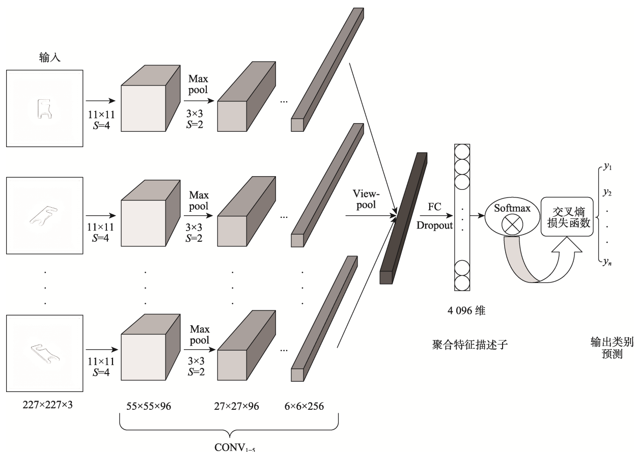
图5 基于 MVCNN 优化的全局特征提取网络
