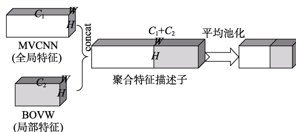
图6 基于特征融合的双尺度特征描述子提取过程
