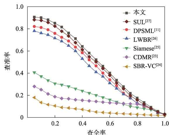
图 7 不同方法的 PR 曲线对比
