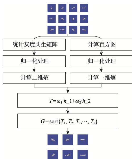
图 2 联合图像熵的最优视图集选取流程
