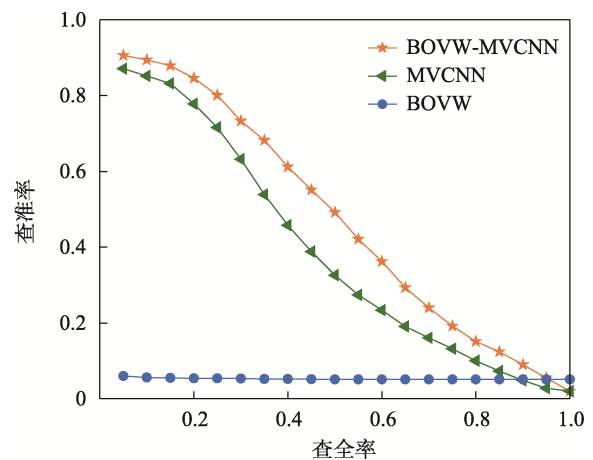
图 9 消融实验的 PR 曲线
