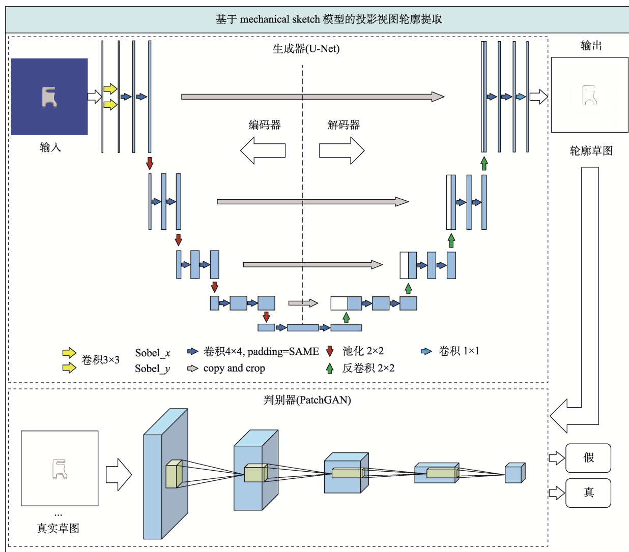
图 3 mechanical sketch 模型结构
