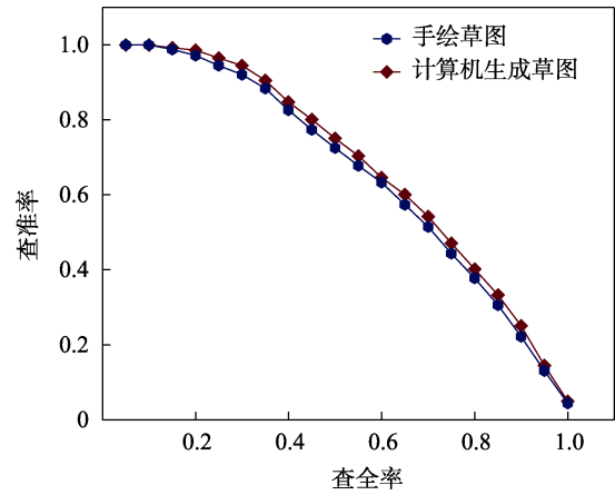
图 8 草图轮廓提取实验的 PR 曲线
