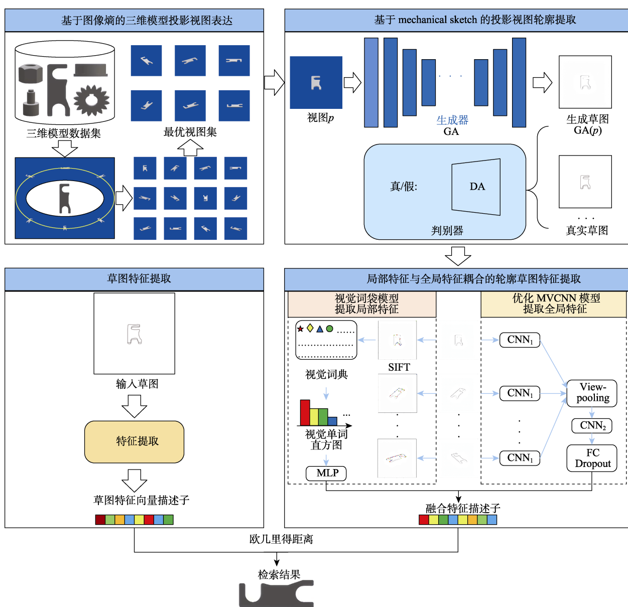
图 1 本文方法框架
