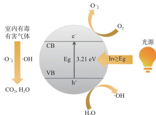
图2 TiO 2 光催化原理示意图
