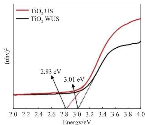
图 12 \text{TiO}_2\text{-US} 与 \text{TiO}_2\text{-WUS} 的 Tauc 图 [47] Fig. 12 Tauc plot of \text{TiO}_2\text{-US} and \text{TiO}_2\text{-WUS} [47]
