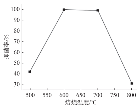
图 6 Li-TiO 2 抗菌材料在不同焙烧温度下对大肠杆菌抗菌性能的影响 [31]
