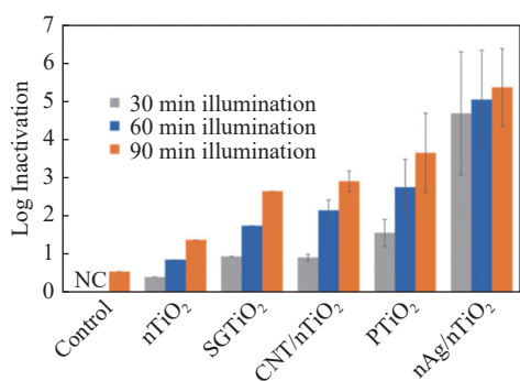
图 8 MS2 噬菌体在接触 30 min、60 min 和 90 min 光触媒 (nTiO 2 、SGTiO 2 、CNT/nTiO 2 、PTiO 2 、nAg/nTiO 2 ) 后的失活实验 (“NC”代表“未收集”) [35]
