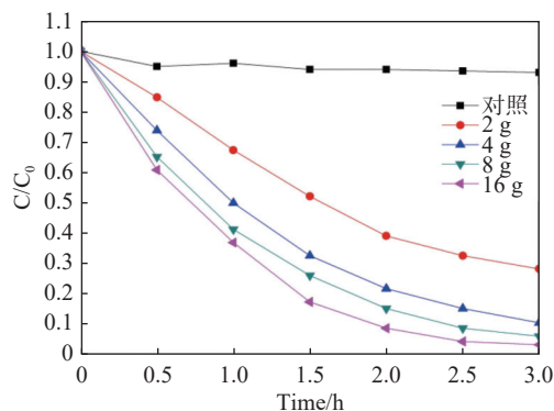
图 9 不同 TiO 2 负载量下 H 2 S 的脱除速率 [36]
