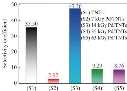
图5 材料对硝酸盐的选择性系数 [25]
