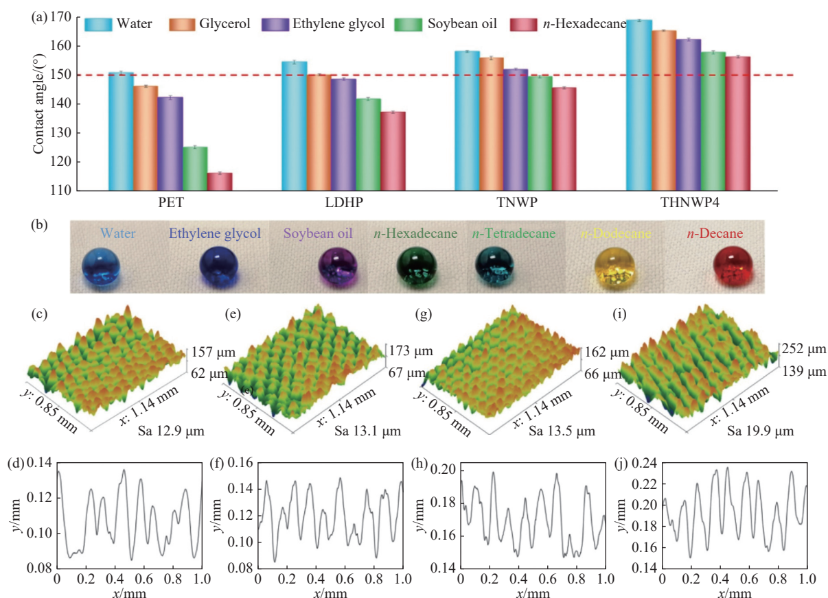
图 10 (a) 不同织物样品上液滴的接触角(CA); (b) THNWP4 表面沉积的彩色液滴照片; 氟化处理的(c)~(d)PET、(d)~(h) LDHP、(e)~(i) TNWP 和(f)~(j) THNWP4 样品的 3D 形貌及表面粗糙度曲线 [40]
