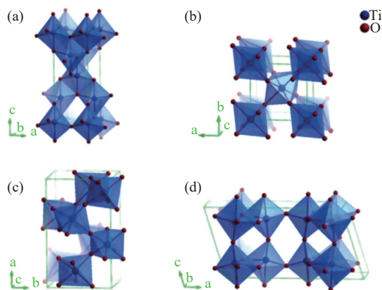
图1 不同晶型 TiO 2 的晶体结构 [10] 。(a)锐钛矿;(b)金红石;(c)板钛矿;(d)特殊结构介孔 TiO 2
