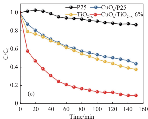
图 11 不同光触媒在相对湿度(RH)为 40% 条件下的光催化性能 [42]
