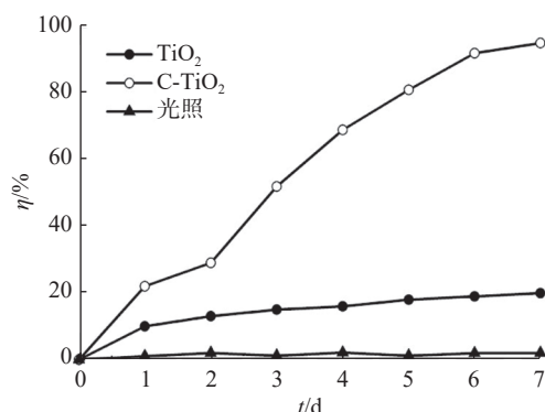
图3 C-TiO 2 和 TiO 2 光触媒对甲醛的去除率(甲醛初始浓度 0.5 μg/L) [17]
