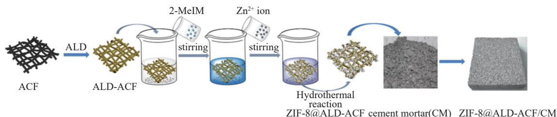
图 13 基于水泥的复合材料制备工艺 [50]
