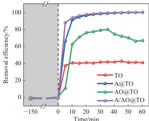
图4 不同样品(TO, A@TO, AO@TO, A/AO@TO)在紫外光( \lambda = 254 nm)下的甲苯去除效率 [22]
