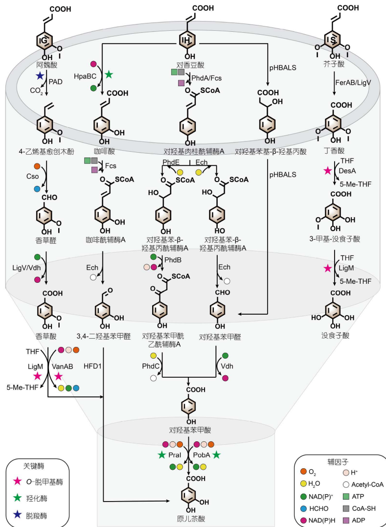
图 2 木质素“生物漏斗”路线生产芳香平台化合物。H型芳香族单体(如对香豆酸)可通过辅酶A依赖的 \beta -氧化途径、CoA依赖的非 \beta -氧化途径及CoA非依赖途径转化为原儿茶酸; G型芳香族单体(如阿魏酸)可通过非氧化脱羧途径转化为原儿茶酸; S型芳香族单体(如丁香酸)可转化为没食子酸。路线中的O-脱甲基酶、羟化酶、和脱羧酶分别用梅红色、绿色和蓝色五角星标示。辅助因子以靠近各酶的彩色圆点标示。PAD, 阿魏酸脱羧酶; Cso2, 类胡萝卜素裂解加氧酶; LigV/Vdh, 香草醛脱氢酶; VanAB, 香草酸O-脱甲基酶; LigM, 香草酸O-脱甲基酶; HpaBC, 4-羟基苯乙酸3-单加氧酶; Fcs, 酰基-辅酶A合成酶; Ech, 烯酰辅酶A水合酶; HFD1, 十六烯醛脱氢酶; PhdA, p -羟基肉桂酰-辅酶A合成酶; PhdB, 3-羟基酰基-辅酶A脱氢酶; PhdC, 3-氧代酰基-辅酶A酮水解酶; PhdE/Ech, 烯酰辅酶A水合酶; Vdh, 香草醛脱氢酶; Pral/PobA, 对羟基苯甲酸羟化酶; pHBALS, p -羟基苯甲醛合成酶; FerA, 阿魏酰-辅酶A合成酶; FerB, 阿魏酰-辅酶A水合酶/裂合酶; LigV, 香草醛脱氢酶; DesA, O-脱甲基酶; LigM, 香草酸/3-O-甲基没食子酸O-脱甲基酶
