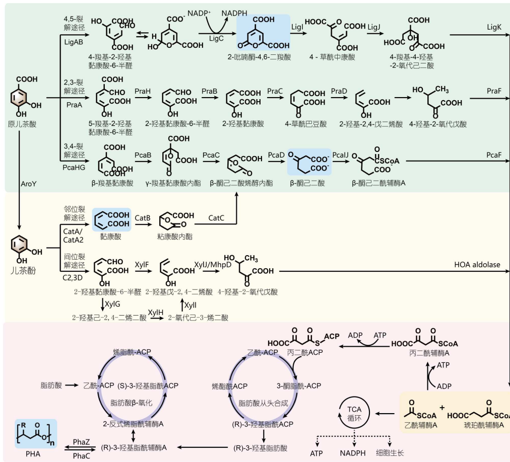
图 4 木质素芳香环开环路线生产高附加值产品。利用特定微生物固有的木质素分解能力，通过芳香环开环途径将异质性木质素衍生物转化为生物塑料及其他高价值化学品。原儿茶酸的芳香环裂解途径包括4,5-裂解途径、2,3-裂解途径和3,4-裂解途径。原儿茶酸的裂解途径以绿色底纹标示。邻苯二酚的邻位裂解途径包括邻位裂解途径和间位裂解途径，以黄色底纹标示。其他重要化学品包括2-吡喃酮-4,6-二羧酸、β-酮己二酸、黏康酸、PHA以蓝色底纹标示。LigAB, 原儿茶酸4,5-双加氧酶; LigC, 4-羧基-2-羟基黏康酸-6-半醛脱氢酶; LigI, 2-吡喃酮-4,6-二羧酸水解酶; LigJ, 4-草酰巴豆酸水合酶; LigK, 4-羧基-4-羟基-2-氧代己二酸醛缩酶; PraA, 原儿茶酸2,3-双加氧酶; PraH, 5-羧基-2-羟基黏康酸-6-半醛脱羧酶; PraB, 2-羟基黏康酸-6-半醛脱氢酶; PraC, 4-草酰巴豆酸互变异构酶; PraD, 4-草酰巴豆酸脱羧酶; PraF, 4-羟基-2-氧代戊酸醛缩酶; PcaHG, 原儿茶酸3,4-双加氧酶; PcaB, 顺,顺-黏康酸环异构酶; PcaC, 4-羧基黏康酸内酯脱羧酶; PcaD, 3-氧代己二酸烯醇内酯酶; PcaIJ, 3-氧代己二酰辅酶A转移酶; PcaF, 4-羟基-2-氧代戊酸醛缩酶; AroY, 原儿茶酸脱羧酶; CatA/CatA2, 邻苯二酚1,2-双加氧酶; CatB, 顺,顺-黏康酸环异构酶; CatC, 黏康酸环异构酶; C2,3D, 邻苯二酚2,3-双加氧酶; XylF, 2-羟基黏康酸半醛水解酶; XylJ/MhpD, 2-氧代戊-4-烯酸水合酶; XylG, 2-羟基黏康酸半醛脱氢酶; XylH, 2-羟基黏康酸互变异构酶; XylI, 2-氧代-3-己烯二酸脱羧酶; HOA aldolase, 4-羟基-2-氧代戊酸醛缩酶
