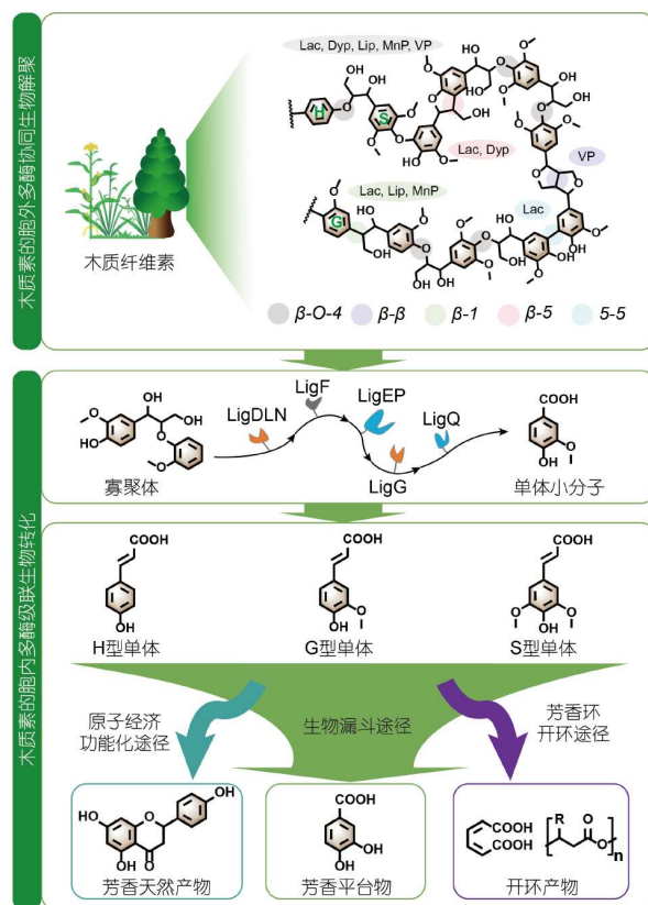
图 1 木质素生物解聚与转化通路. 木质素中 \beta -O-4、 \beta - \beta 、 \beta -1、 \beta -5、5-5键在木质素降解酶胞外多酶协同作用下断裂, 使木质素实现生物解聚. 解聚得到的寡聚体通过胞内多酶级联生物转化成为芳香族小分子. 小分子通过生物漏斗途径、原子经济功能化途径和芳香环开环途径进行胞内多酶级联生物转化, 分别生产出芳香平台物、芳香天然产物和开环产物. 图中运用灰色、紫色、绿色等不同颜色标记不同木质素降解酶系对应断裂木质素中的不同键型. 图中以木质素二聚体 \beta -O-4模型化合物愈创甘油醚- \beta -愈创甘油醚为代表展示木质素寡聚体胞内多酶级联生物转化过程. Lac, 漆酶; Dyp, 染料脱色过氧化物酶; Lip, 木质素过氧化物酶; MnP, 锰过氧化物酶; VP, 多功能过氧化物酶
