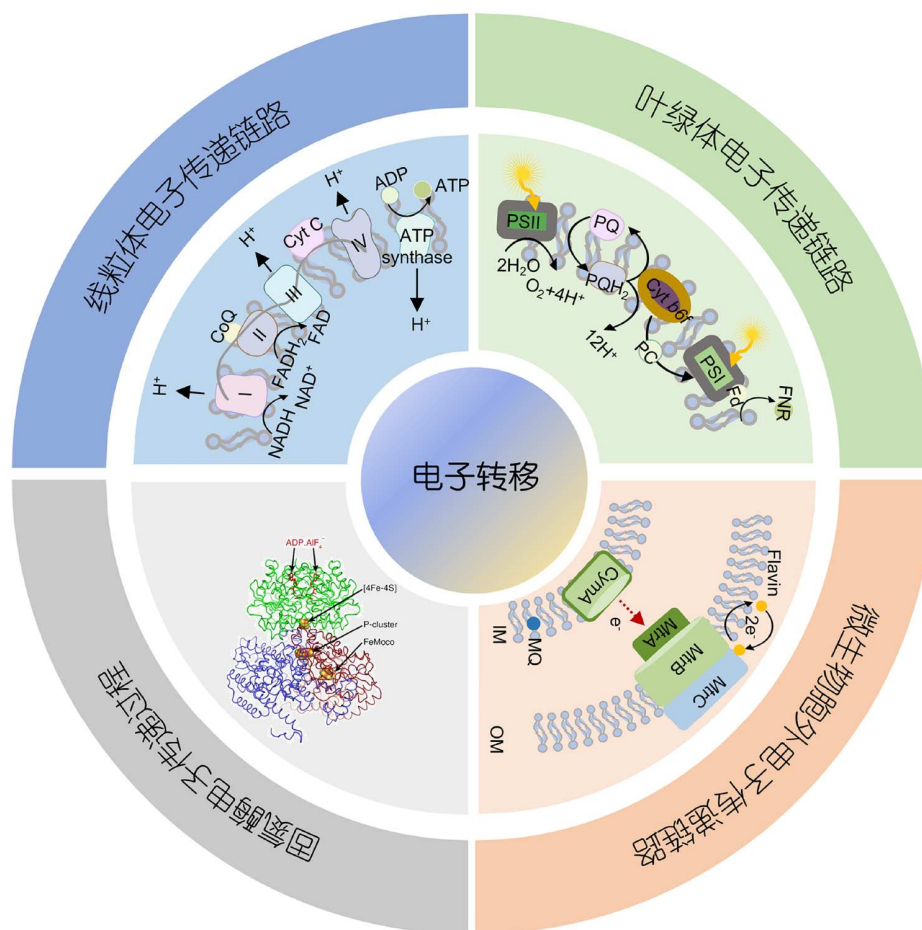
图 1 生命系统中的电子转移过程示意图(图片修改自文献[45], 已获American Chemical Society版权许可)
