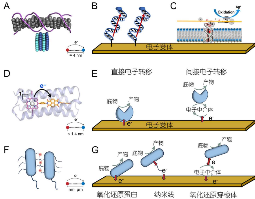
图 2 基于DNA、蛋白质和电活性菌的生物电子界面构建策略。A~C: DNA电荷传输性质与电子界面构建策略(修改自文献[70,72,75]。文献[70,75]已获American Chemical Society版权许可, 文献[72]为开放获取); D: 蛋白质内部电子转移示意图(修改自文献[97], 已获American Chemical Society版权许可); E: 蛋白质与电极界面间的电子转移策略; F: 电活性菌的EET过程示意图; G: 从左至右分别为电活性菌通过细胞色素蛋白介导的DET、通过导电菌毛介导的DET以及通过电子传递中介体介导的IET
