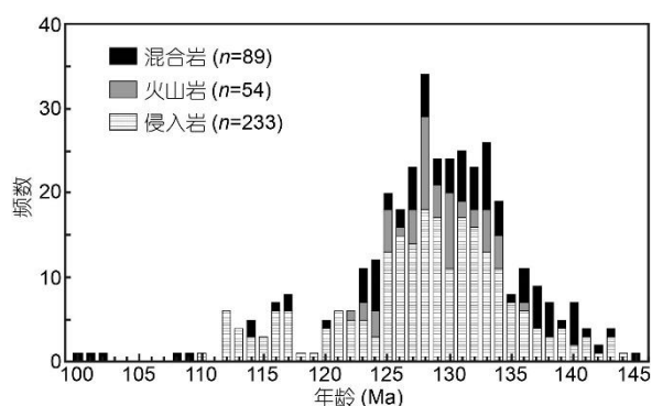
图 12 大别造山带晚中生代岩浆活动和混合岩化作用年龄汇总。侵入岩年龄据 Wang 等 (2007)、Xu 等 (2007)、He 等 (2011) 及其引文、Gao 等 (2016a) 及其引文、Zhao 等 (2017) 及其引文、Yan 等 (2021) 及其引文、Huang 等 (2024) 及其引文、Wang 等 (2024) 及其引文；火山岩年龄据王岳军等 (2002)、Fan 等 (2004)、Dai 等 (2016)、Gao 等 (2016b) 及其引文、Zhu 等 (2017) 及其引文；混合岩年龄据 Wu 等 (2007)、Wang 等 (2013) 及其引文、Xu 和 Zhang (2017) 及其引文、王勇生等 (2018) 及其引文、Xia 等 (2023) 及其引文、Lei 等 (2024) 及其引文、Wang 等 (2025) 及其引文
