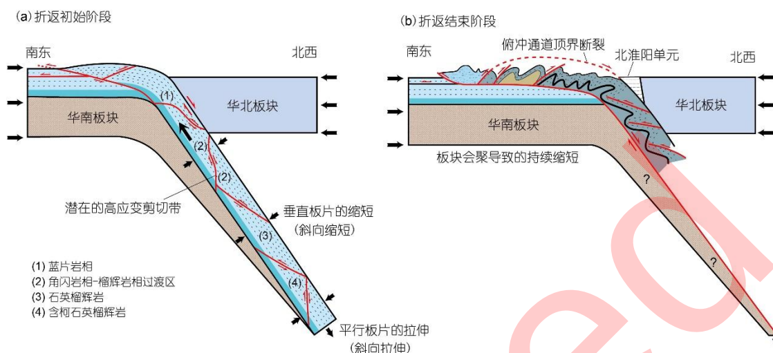
图9 大别造山带俯冲板片解耦及多板片折返示意图，据Hacker等（2000）修改
