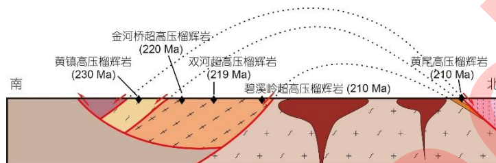
图 5 大别造山带中南部的堆叠岩片及变质年龄的穿时性特征，据 Wang 等（2008）修改。年龄数据为高压-超高压变质岩折返至地壳底部的锆石 U-Pb 年龄结果，来源：Ayers 等，2002；Liu 等，2006；Leech 等，2013 及其引文。图例同图 2。
