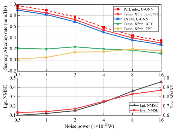
图 11 (网络版彩图) 安全 AirComp 性能随噪声功率的变化。
