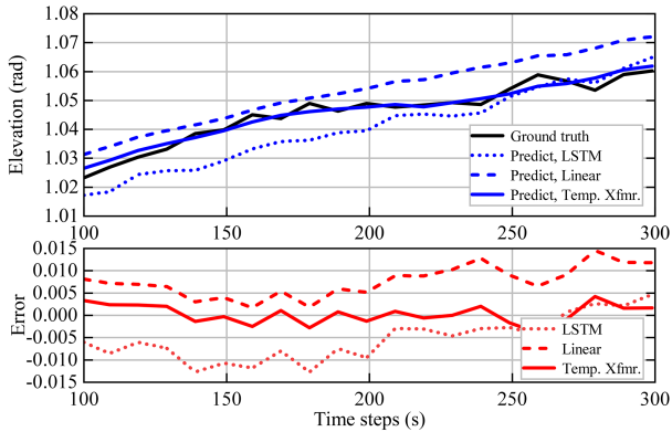
图 7 (网络版彩图) 星间链路俯仰角的预测。
