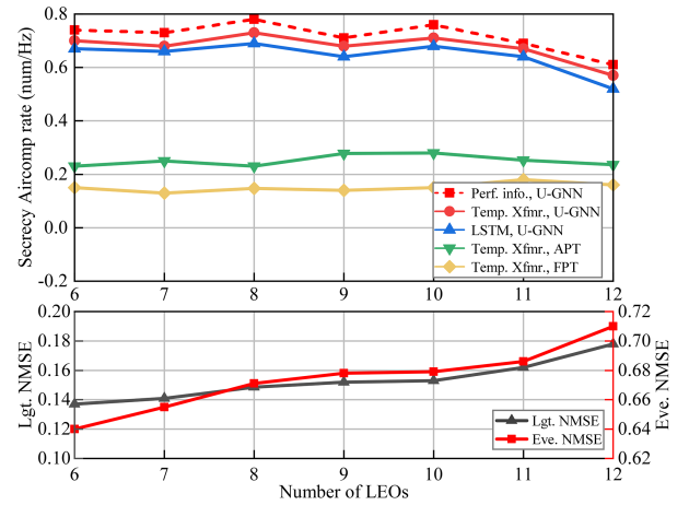
图 8 (网络版彩图) 安全 AirComp 性能随 LEO 卫星数的变化。
