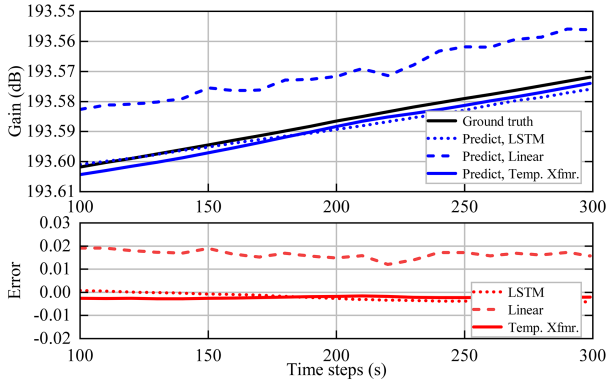
图 5 (网络版彩图) 星间链路增益的预测。
