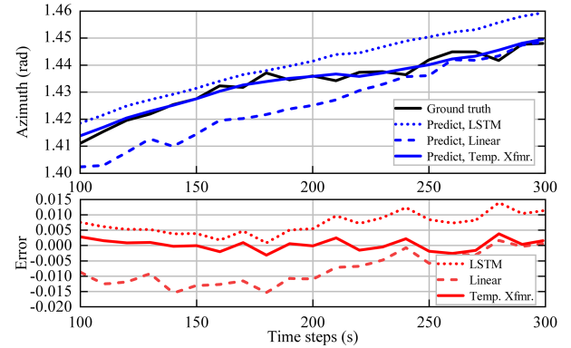
图 6 (网络版彩图) 星间链路方位角的预测。
