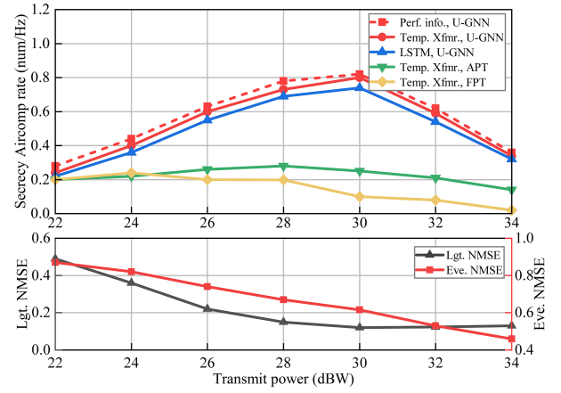
图 10 (网络版彩图) 安全 AirComp 性能随最大发射功率的变化。
