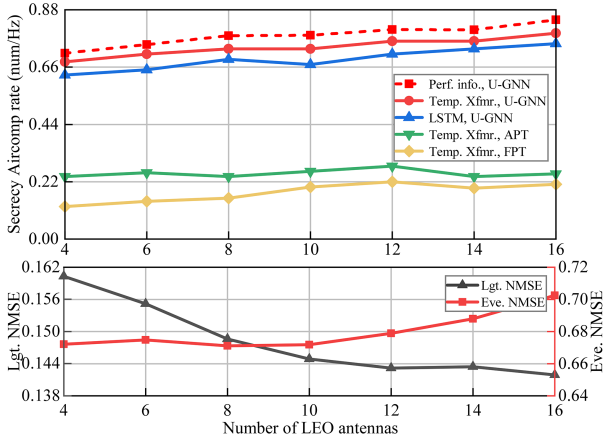
图 9 (网络版彩图) 安全 AirComp 性能随 LEO 卫星天线数的变化。
