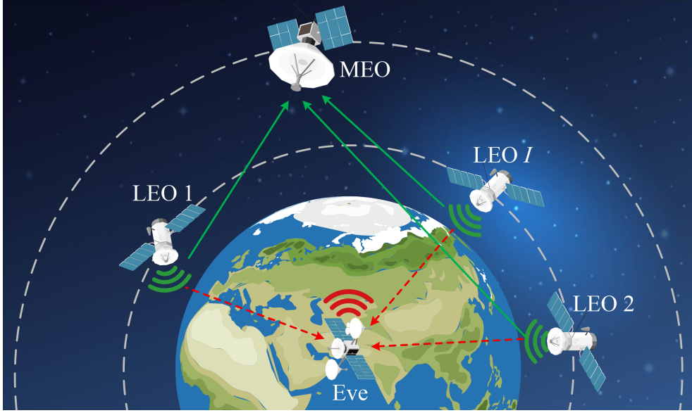
图 1 (网络版彩图) 系统模型.
