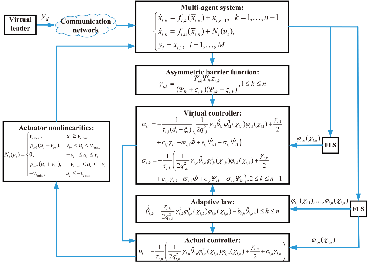
图3 (网络版彩图) 控制方法结构框图.
