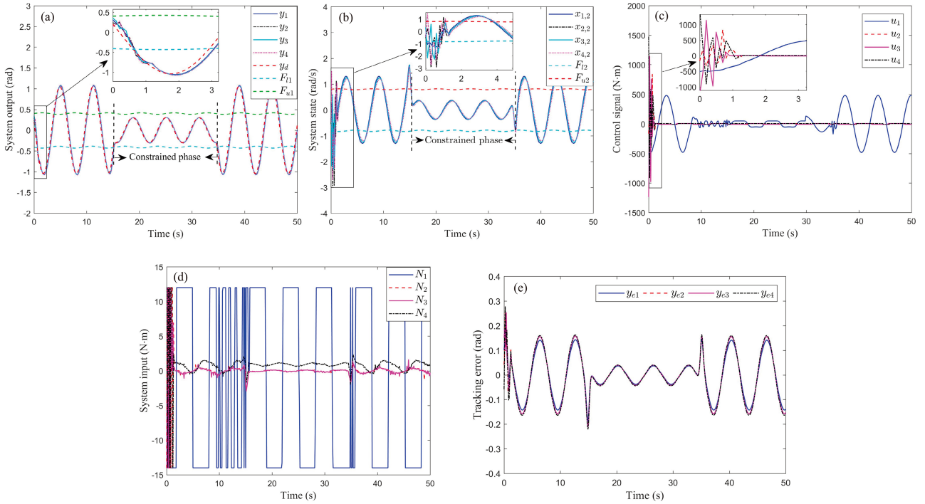
图6 (网络版彩图) 扭摆系统仿真结果. (a) 扭摆输出 y_i ; (b) 扭摆状态 x_{i,2} ; (c) 扭摆控制信号 u_i ; (d) 扭摆输入 N_i ; (e) 扭摆跟踪误差 y_{ei} .
