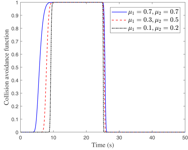
图 1 (网络版彩图) 避撞函数 \Phi(t) 的演变轨迹.
