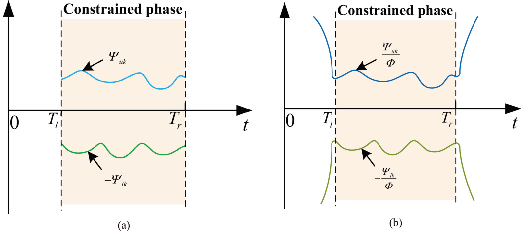
图 2 (网络版彩图) 避撞函数 \Phi(t) 作用下的约束形式. (a) 约束 -\Psi_{lk} < z_{i,k} < \Psi_{uk} 示意图; (b) 约束 -\frac{\Psi_{lk}}{\Phi} < z_{i,k} < \frac{\Psi_{uk}}{\Phi} 示意图.
