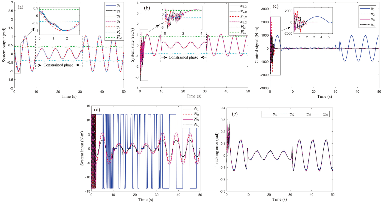
图 5 (网络版彩图) 机器人系统仿真结果. (a) 系统输出 y_i ; (b) 系统状态 x_{i,2} ; (c) 控制信号 u_i ; (d) 系统输入 N_i ; (e) 跟踪误差 y_{ei} .
