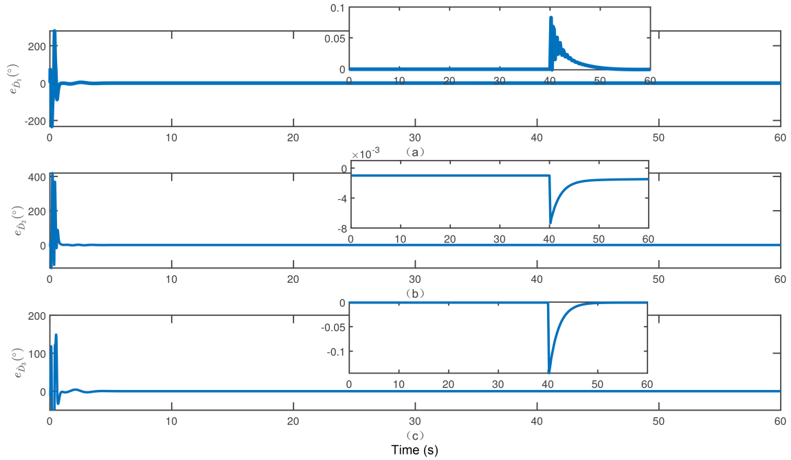
图 3 (网络版彩图) 故障估计误差曲线.
