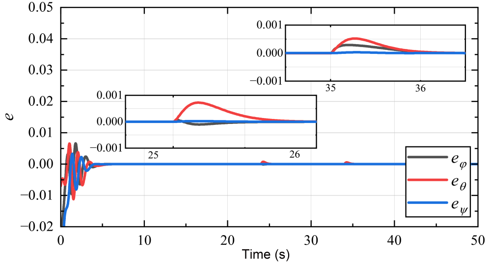
图 5 (网络版彩图) 姿态角跟踪误差曲线.
