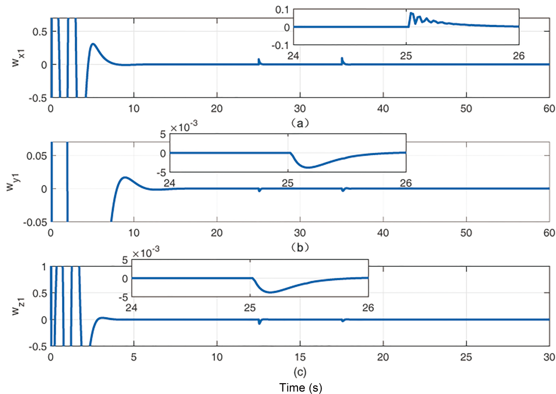
图 6 (网络版彩图) 姿态角速度变化曲线.
