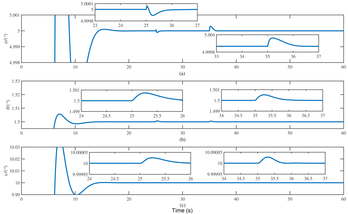
图 4 (网络版彩图) 发生执行器故障时的运载火箭姿态角变化曲线.
