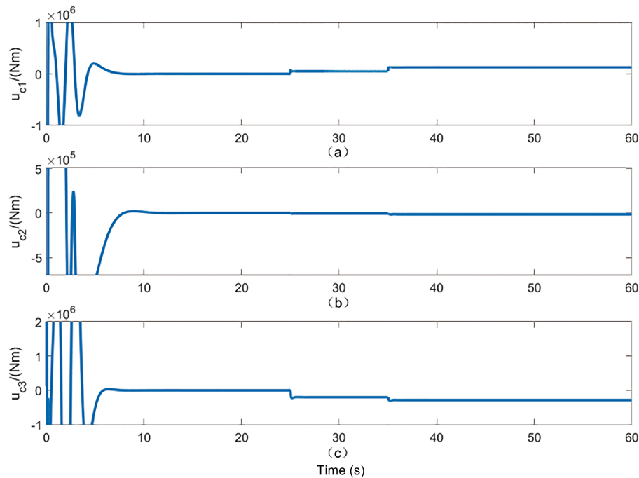
图 7 (网络版彩图) 控制输入 u_c .
