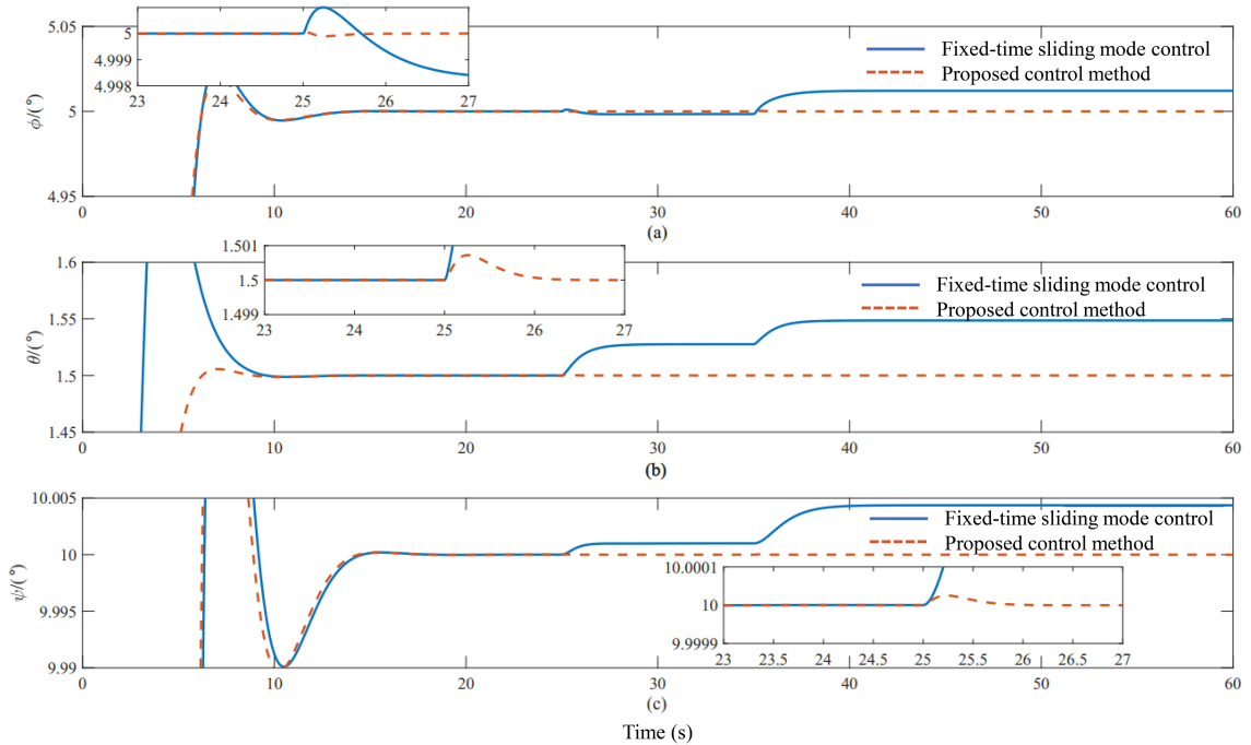
图 9 (网络版彩图) 姿态角对比曲线.
