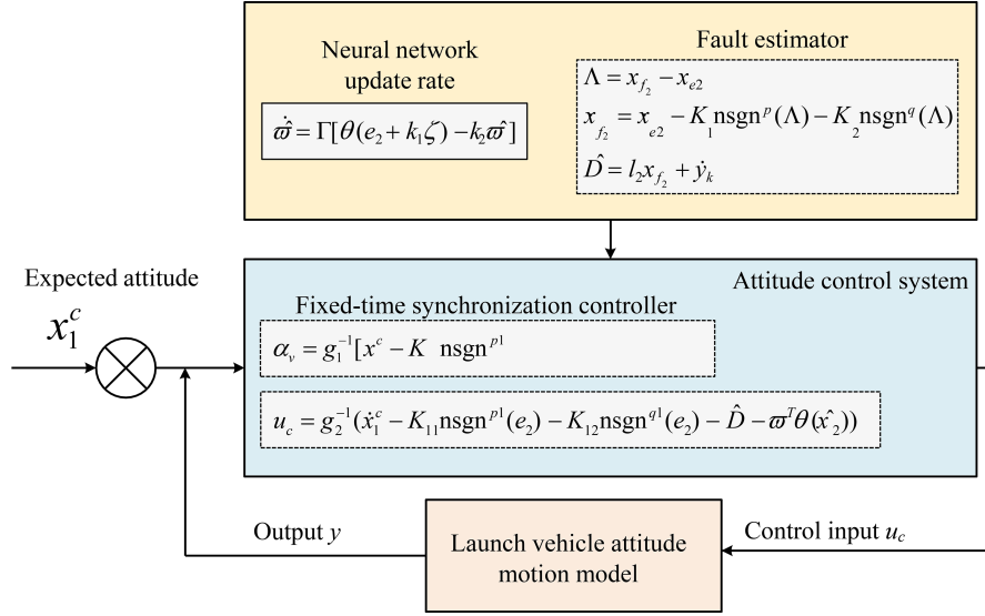
图 2 (网络版彩图) 基于复合学习和固定时间同步的运载火箭姿态容错控制系统图.
