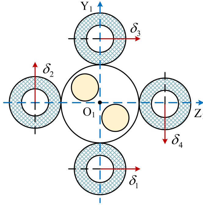
图 1 (网络版彩图) 运载火箭发动机布局示意图.
