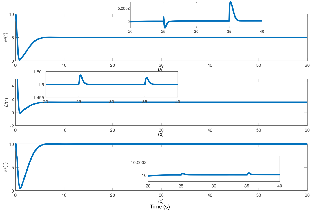
图 8 (网络版彩图) 采用本文方法后的运载火箭姿态角变化曲线.
