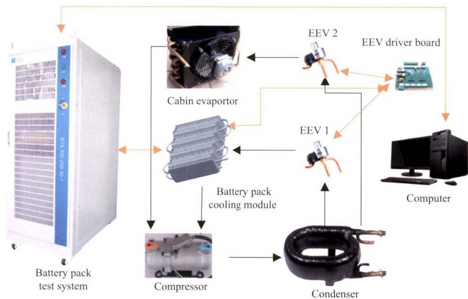
图 6 集成热管理系统原理图 [64]
